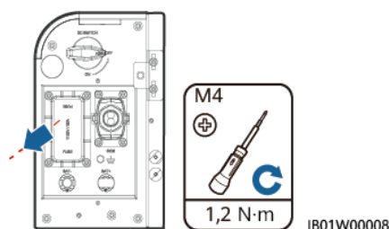
Rysunek 11-1 Zdejmowanie przykręcaniej osłony
