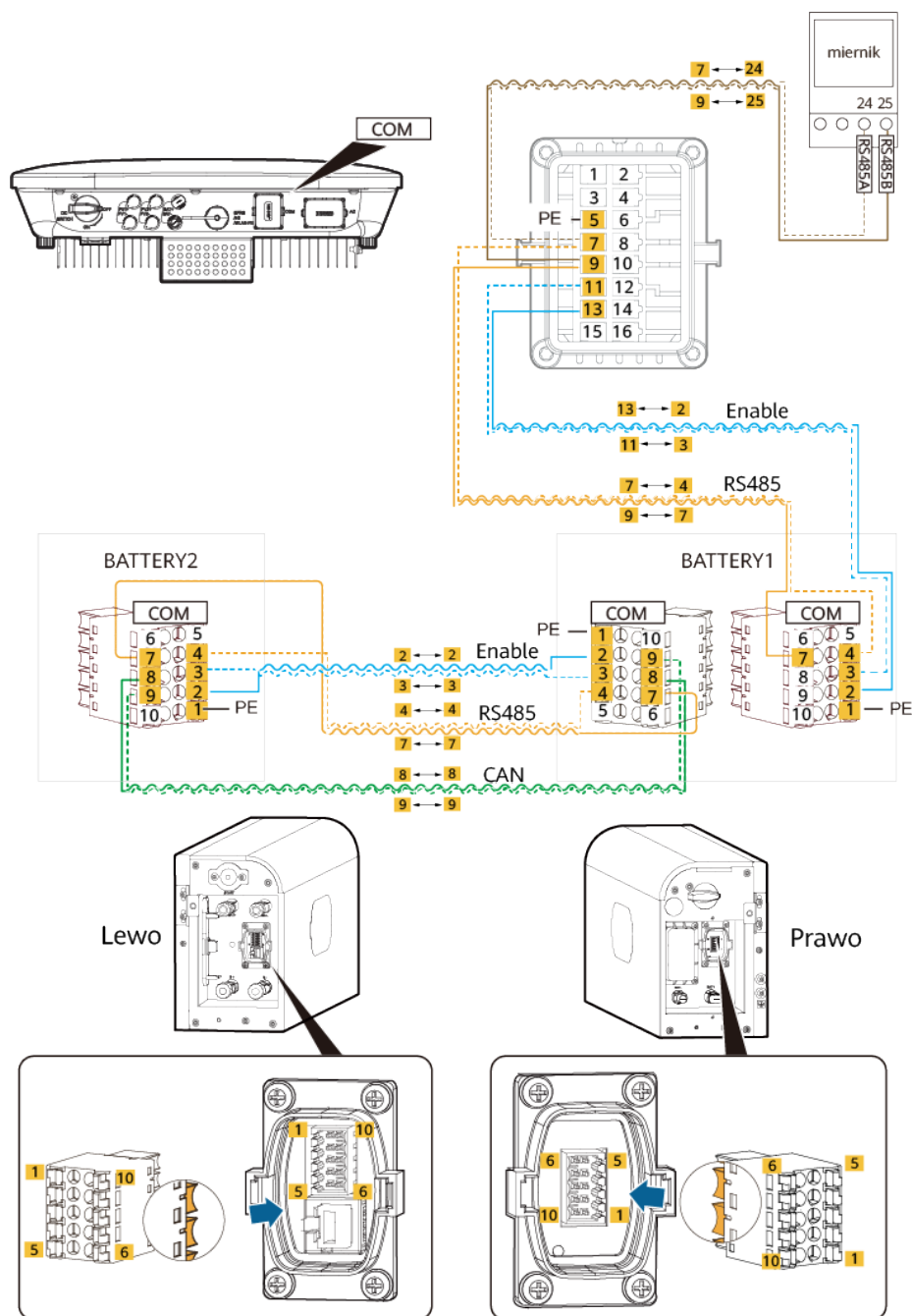
Rysunek 6-7 SUN2000-(3KTL-12KTL)-M1
