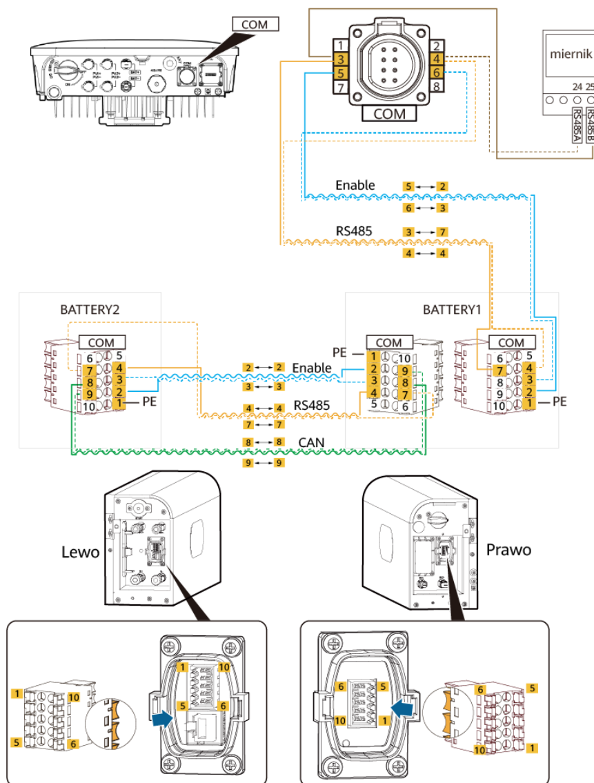
Rysunek 6-6 SUN2000-(2KTL-6KTL)-L1
