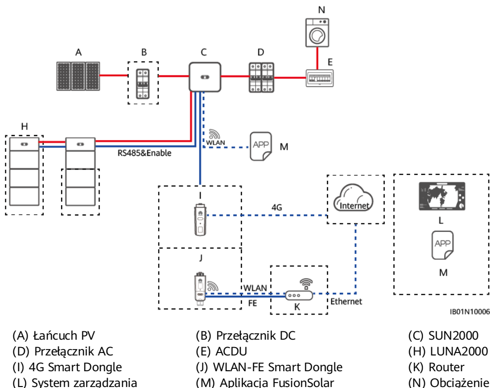
Rysunek 4-15 System magazynowania energii poza siecią (kreskowane pola oznaczają komponenty opcjonalne)
