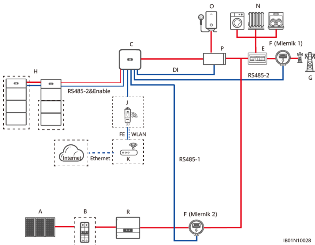
Rysunek 4-17 Połączenie sieciowe z falownikami innej firmy
