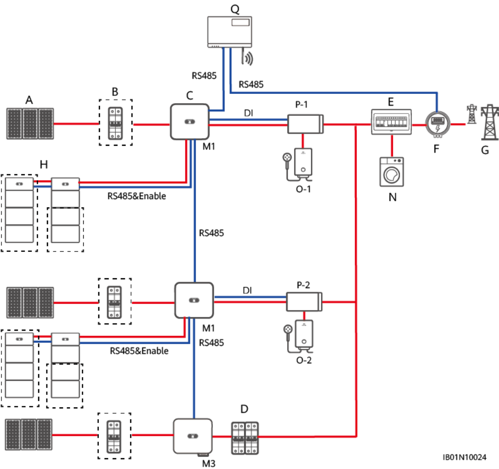
Rysunek 4-12 Połączenie sieciowe dwóch falowników SUN2000-(3KTL-10KTL)-M1 i jednego falownika SUN2000-(20KTL, 29.9KTL, 30KTL, 36KTL, 40KTL)-M3 (kreskowane pola oznaczają komponenty opcjonalne)
