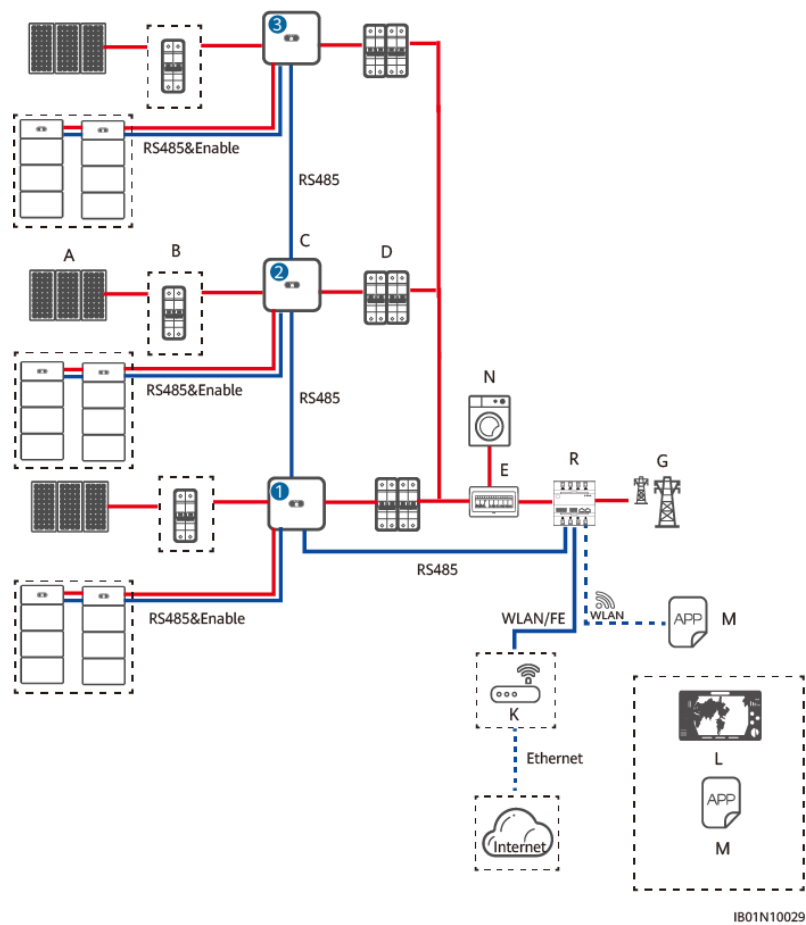
Rysunek 4-4 Połączenie sieciowe EMMA
