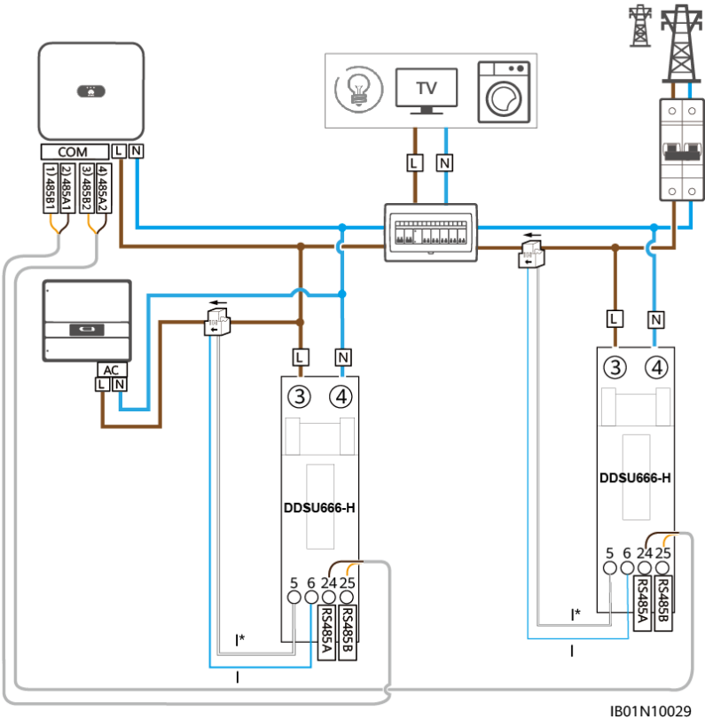
Rysunek 4-18 Połączenia kablowe miernika mocy dla SUN2000-(2KTL-6KTL)-L1
